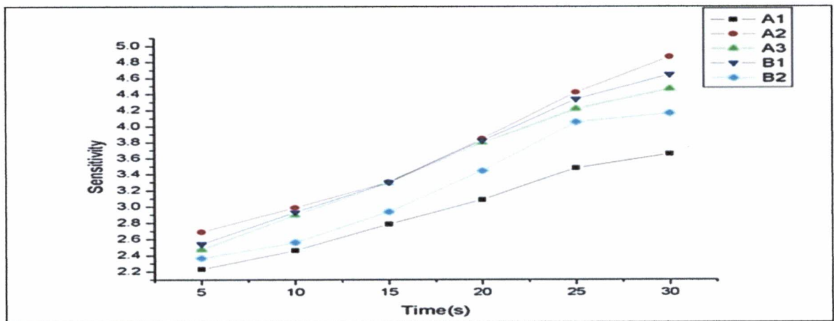
ภาพที่ 1 การตอบสนองต่อแก๊ส Ethanol ของโครงสร้างนาโน CuO
